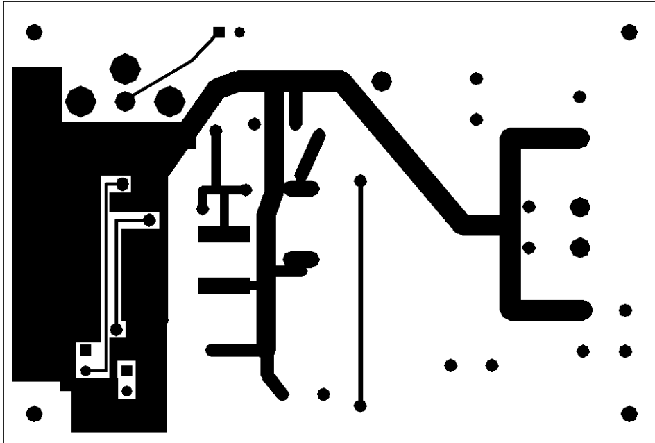
Bottom Layer
