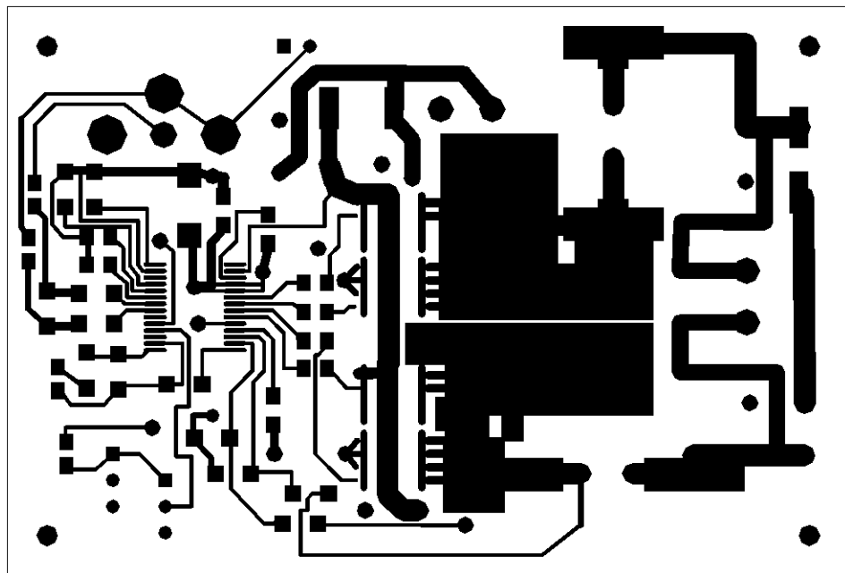
Top Layer
