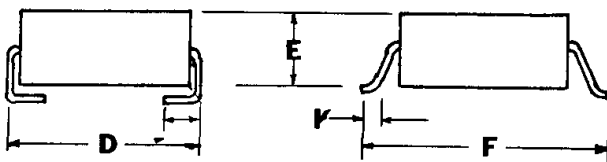
DO-214AA
