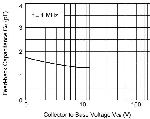
C_{re} - V_{CB}
