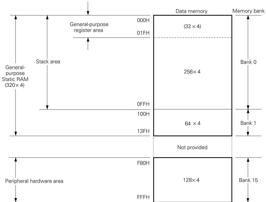
(b) μPD75106, 75104
