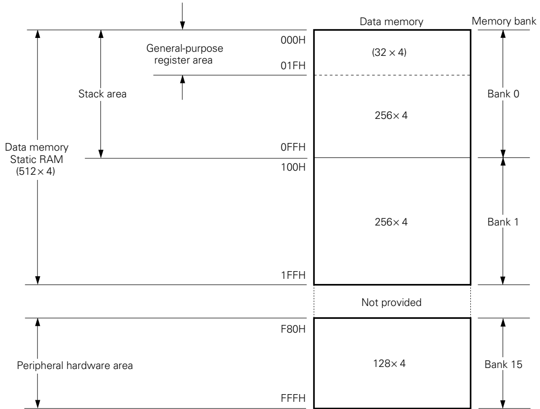
(a) μPD75108
