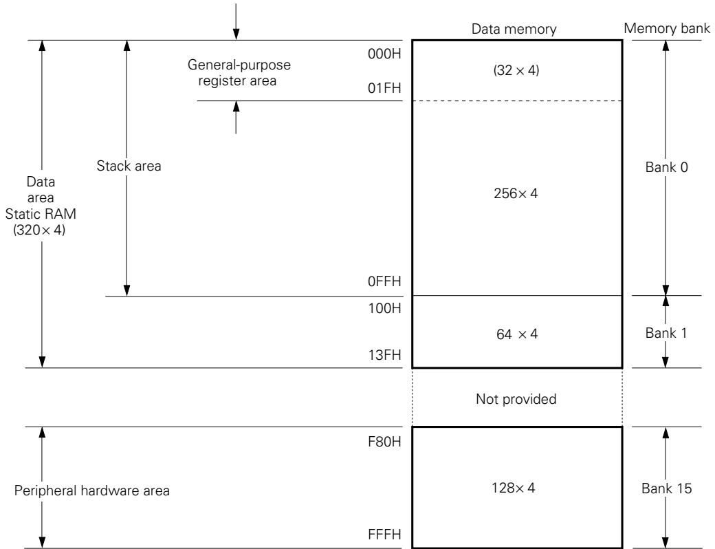
(b) μPD75104A
