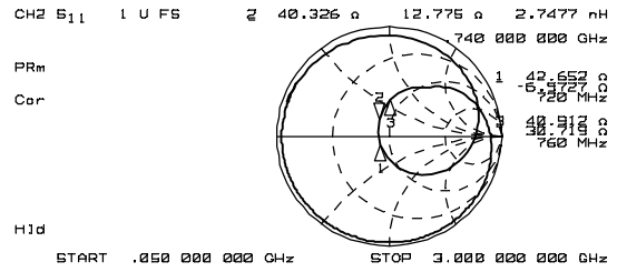
LOIN port Impedance
