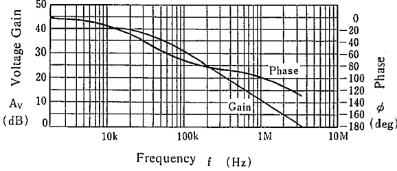
NJM072B/082B
