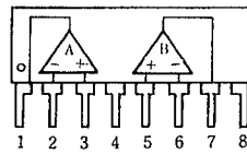
NJM2043L
