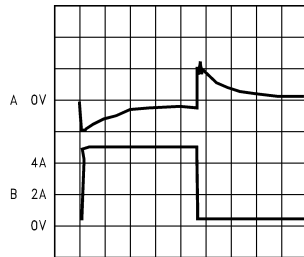
100 \mu sec/Div DS100886-19
