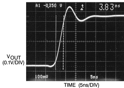
1A. A_V = -1
