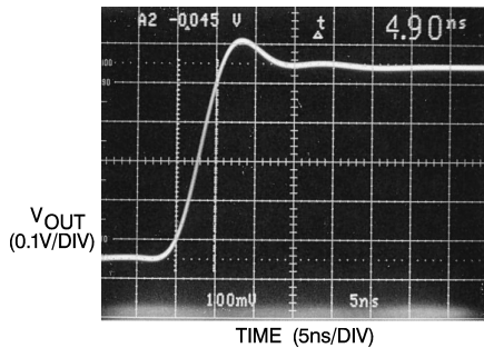
1B. A_V = -5
