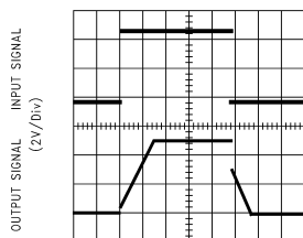
TIME (100 \mu s /Div) DS011422-33
