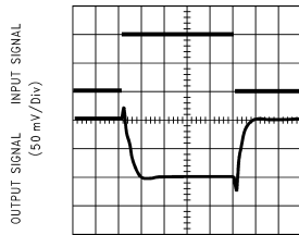
TIME (10 \mu s /Div) DS011422-30
