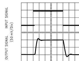
TIME (10 \mu s /Div) DS011422-32
