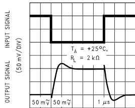
TIME (1 \mu s /DIV) DS011713-84
