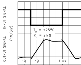
TIME (1 \mu s /DIV) DS011713-81
