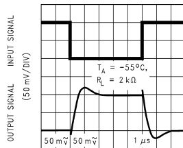
TIME (1 \mu s /DIV) DS011713-85
