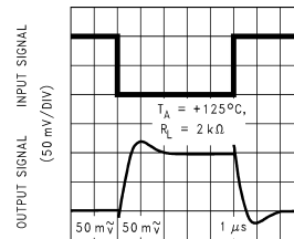
TIME (1 \mu s /DIV) DS011713-83
