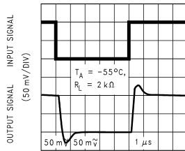
TIME (1 \mu s /DIV) DS012049-64
