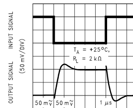
TIME (1 \mu s /DIV) DS012049-69
