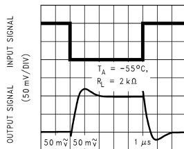
TIME (1 \mu s /DIV) DS012049-70
