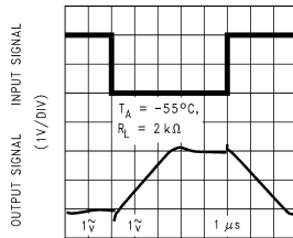
TIME (1 \mu s /DIV) DS012049-67
