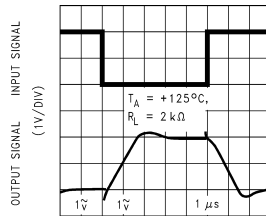
TIME (1 \mu s /DIV) DS012049-65
