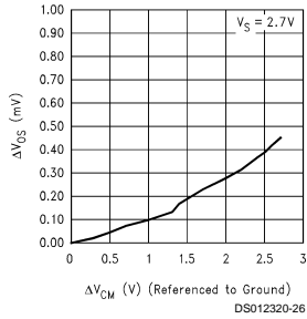
\Delta V_{OS} vs \Delta V_{CM}
