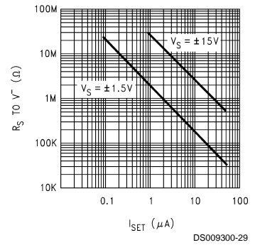
R_{SET} vs I_{SET}
