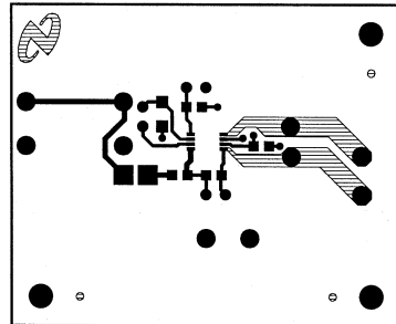
Top Layer
