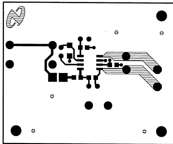
Top Layer
