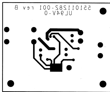
Bottom Layer
