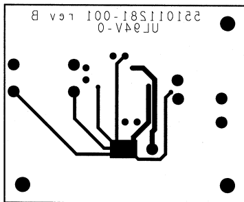
Bottom Layer
