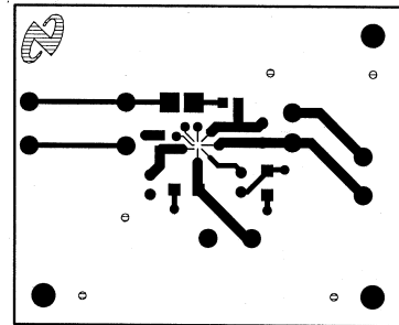
Top Layer
