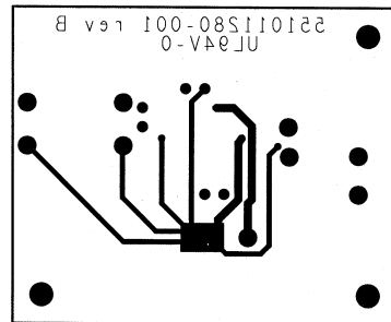
Bottom Layer
