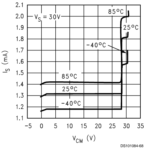
I_S vs. V_{CM}
