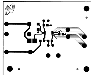
Top Layer
