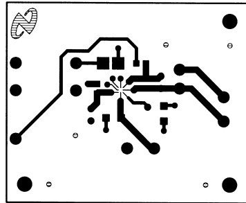
Top Layer
