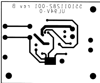
Bottom Layer
