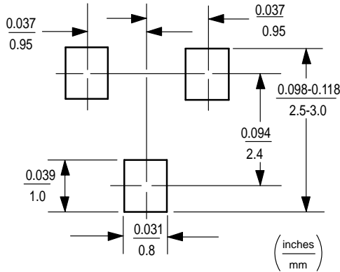
SC-59
