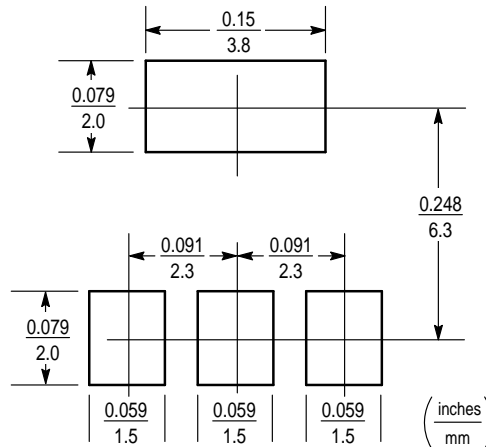
SOT-223
