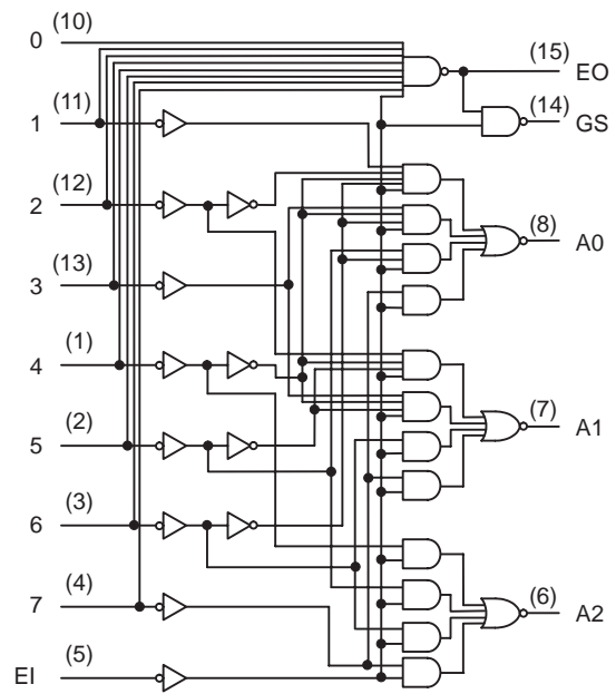
SN74LS148
