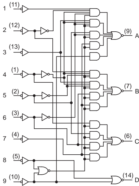
SN74LS147
