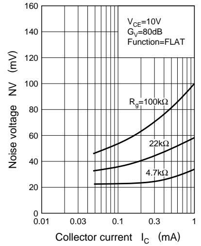
NV — I_C
