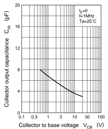
C_{ob} - V_{CB}
