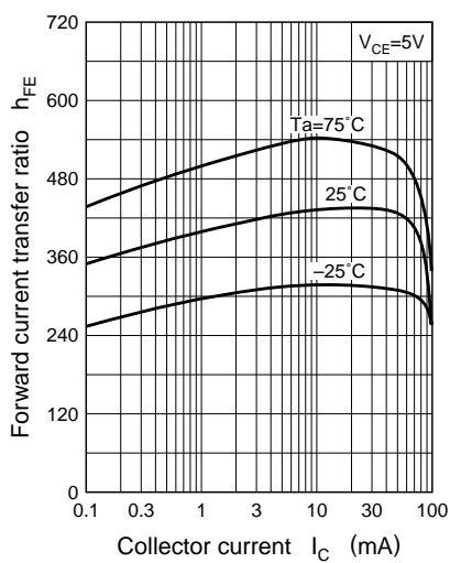
h_{FE} - I_C
