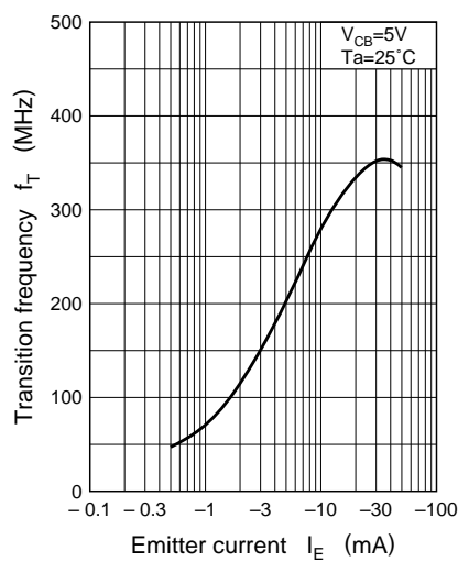
f_T - I_E
