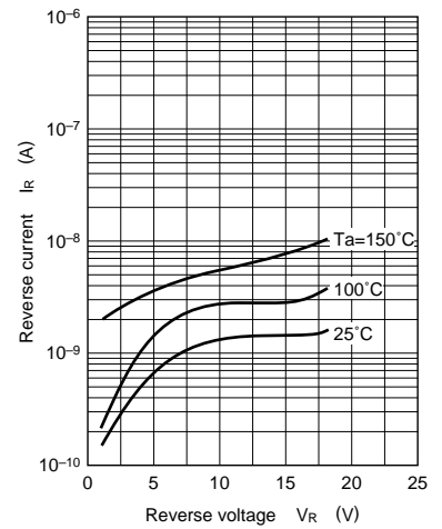
I_R - V_R
