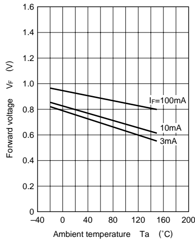
V_F - T_a
