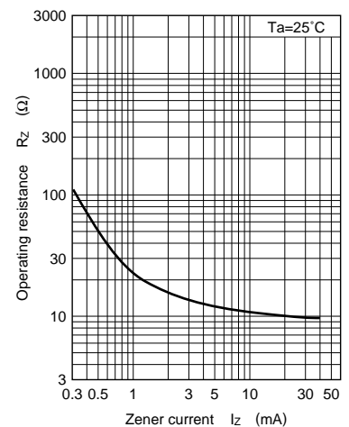
R_Z - I_Z
