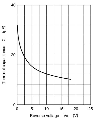
C_t - V_R
