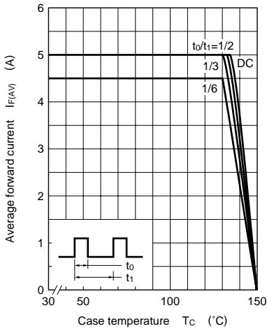
I_{F(AV)} - T_C
