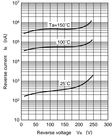
I_R - V_R
