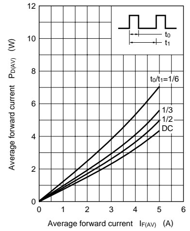
P_{D(AV)} - I_{F(AV)}
