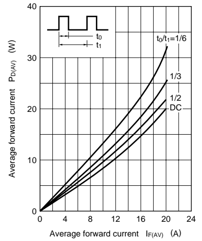
P_{D(AV)} - I_{F(AV)}
