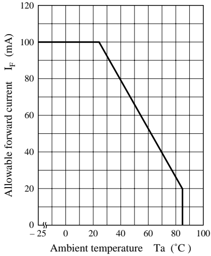
I_F - T_a
