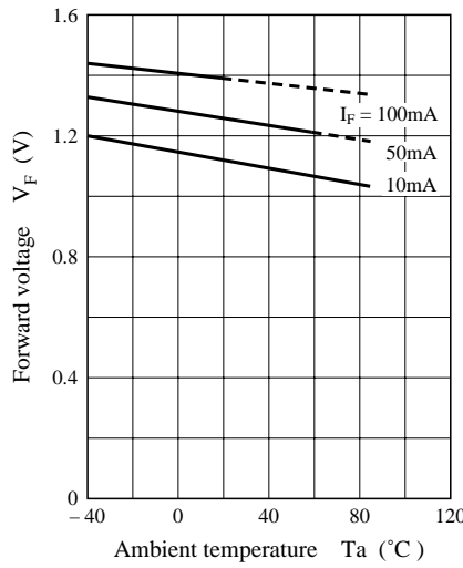
V_F - T_a
