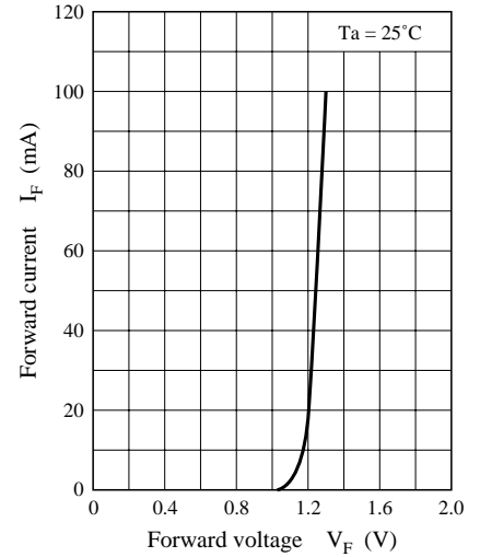
I_F - V_F
