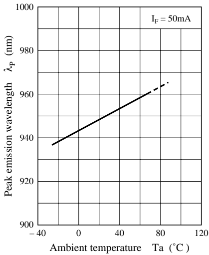
\lambda_p - T_a
