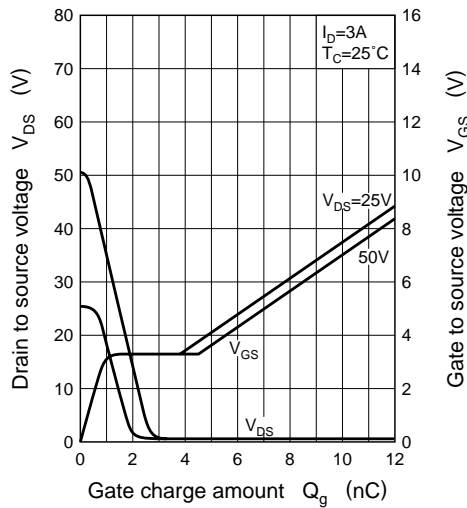
V_{DS}, V_{GS} - Q_g
