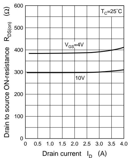
R_{DS(on)} — I_D
