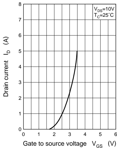
I_D — V_{GS}
