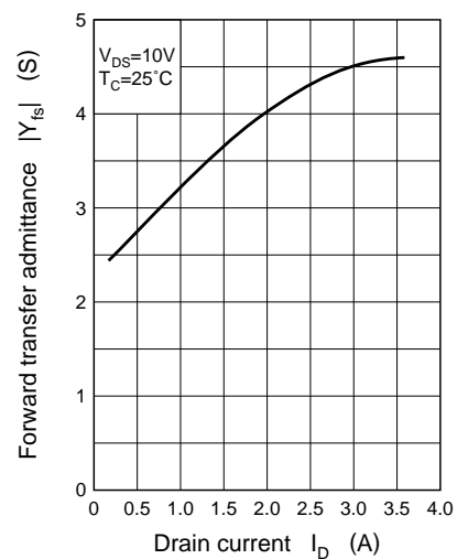
|Y_{fs}| — I_D
