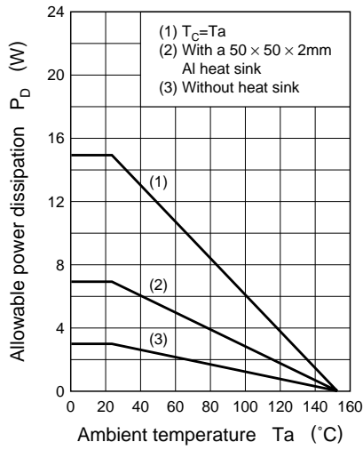
P_D — T_a
