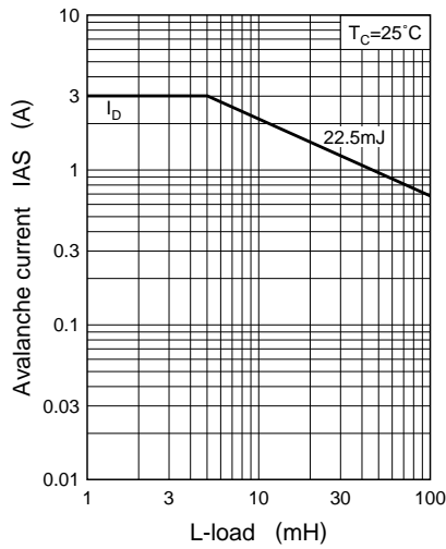
IAS — L-load
