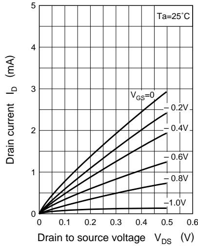
I_D - V_{DS}
