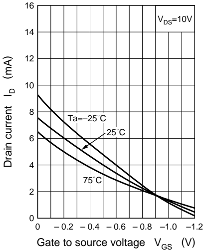
I_D - V_{GS}
