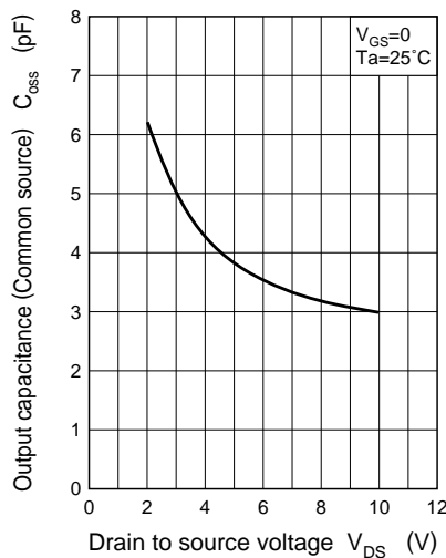
C_{oss} - V_{DS}
