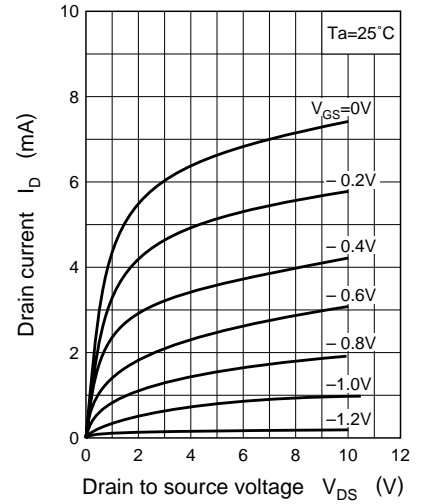
I_D - V_{DS}
