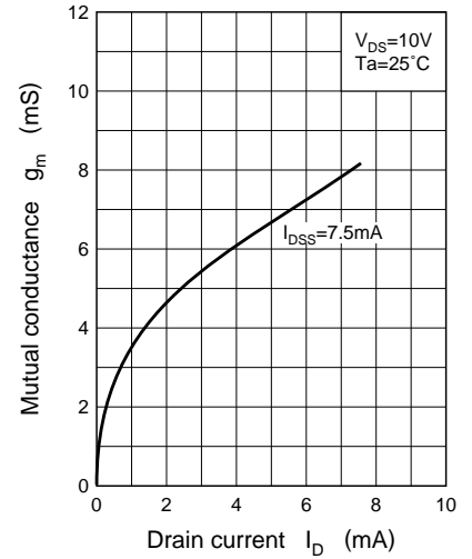
g_m - I_D
