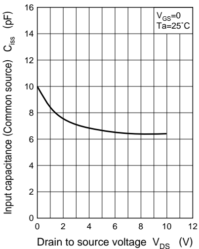
C_{iss} - V_{DS}
