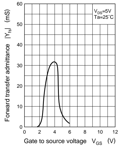
|Y_{fs}| - V_{GS}
