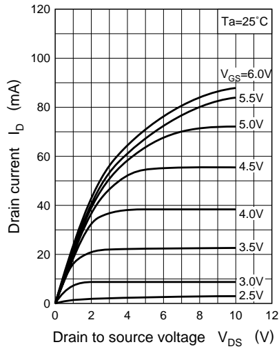
I_D - V_{DS}
