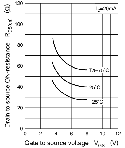
R_{DS(on)} - V_{GS}
