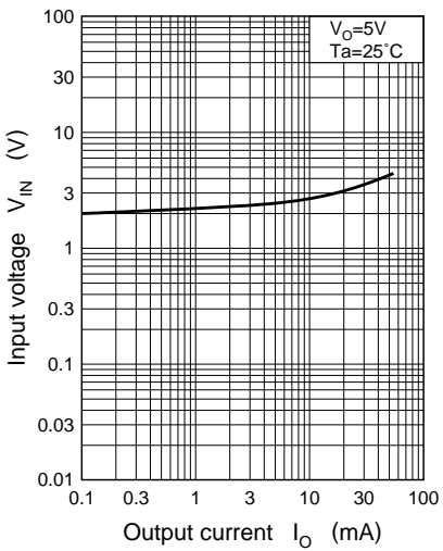
V_{IN} - I_O
