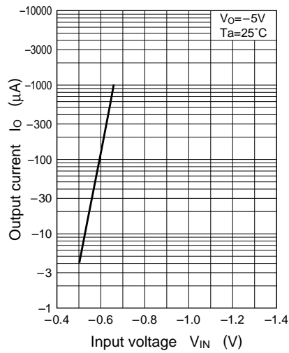
I_O - V_{IN}
