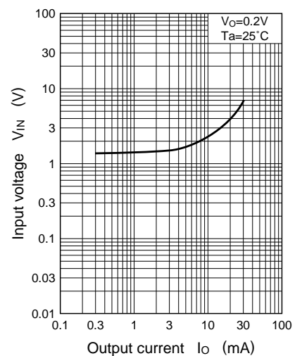
V_{IN} - I_O
