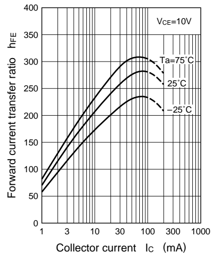
h_{FE} - I_C
