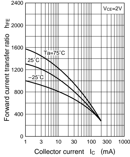
h_{FE} - I_C
