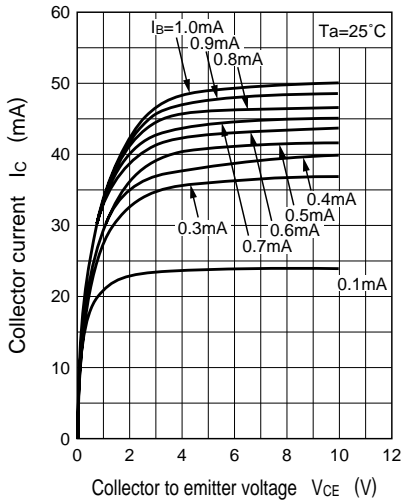
I_C - V_{CE}
