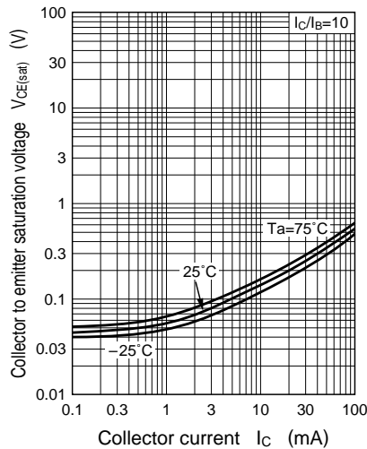
V_{CE(sat)} - I_C
