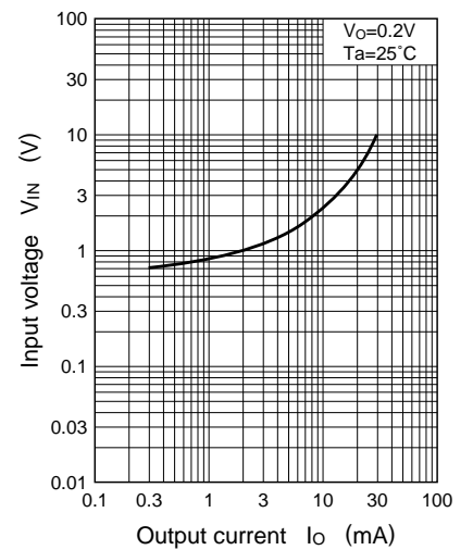
V_{IN} - I_O
