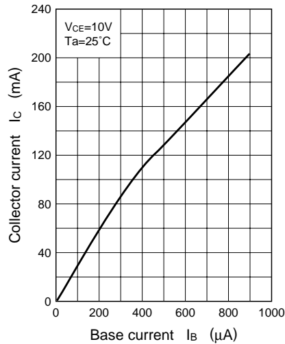
I_C - I_B
