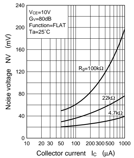
N_V - I_C
