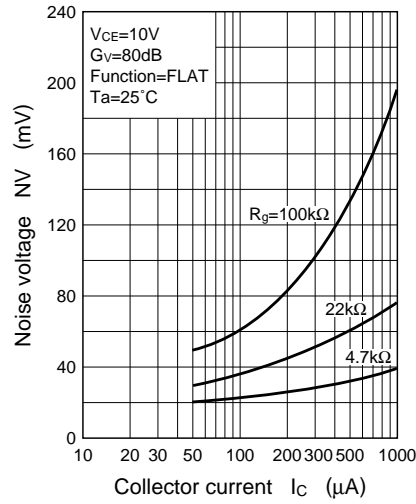
NV - I_C
