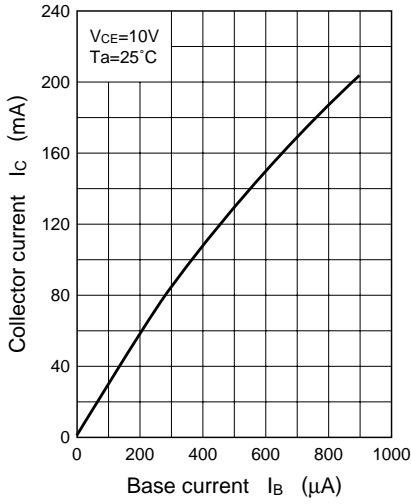
I_C - I_B
