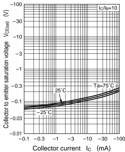
V_{CE(sat)} - I_C
