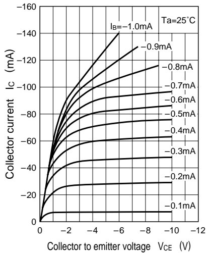
I_C - V_{CE}
