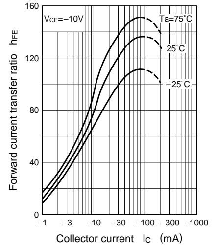
h_{FE} - I_C
