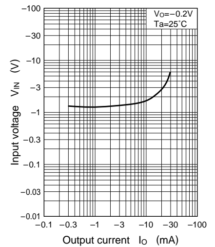
V_{IN} - I_O
