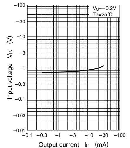
V_{IN} - I_O
