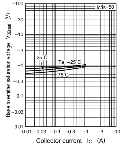
V_{BE(sat)} - I_C
