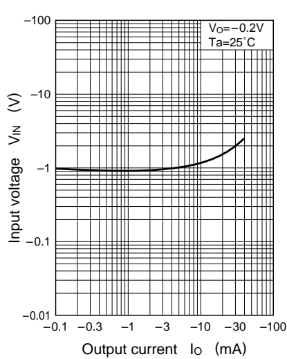
V_{IN} - I_O
