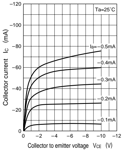
I_C - V_{CE}
