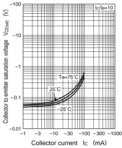
V_{CE(sat)} - I_C
