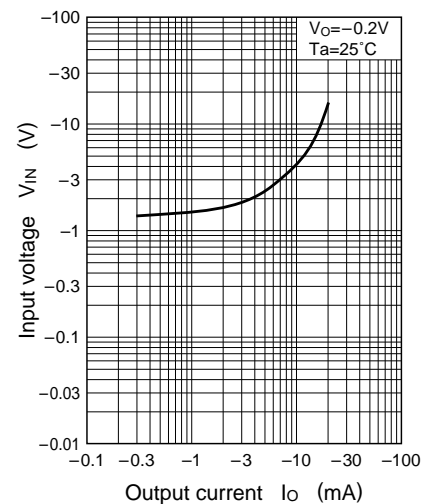
V_{IN} - I_O
