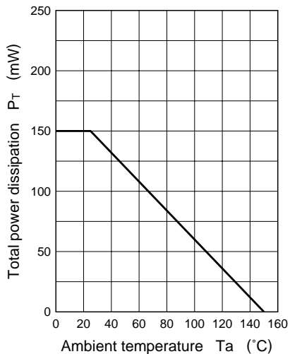
P_T - T_a
