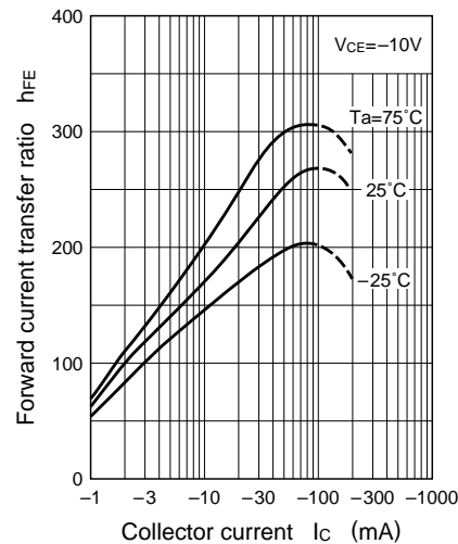
h_{FE} - I_C
