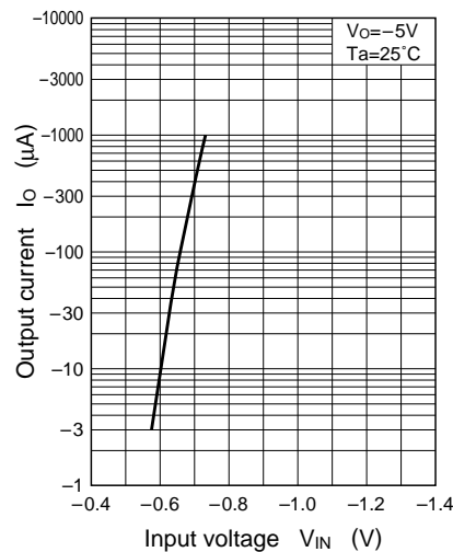
I_O - V_{IN}
