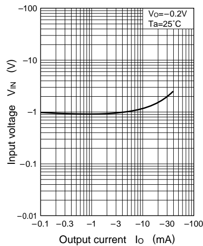
V_{IN} - I_O
