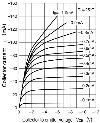
I_C - V_{CE}
