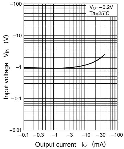
I_O - V_{IN}
