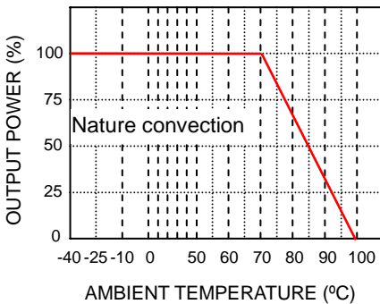
FEC30-24S3P3W (Note 5)
