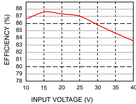
FEC30-24S3P3W
