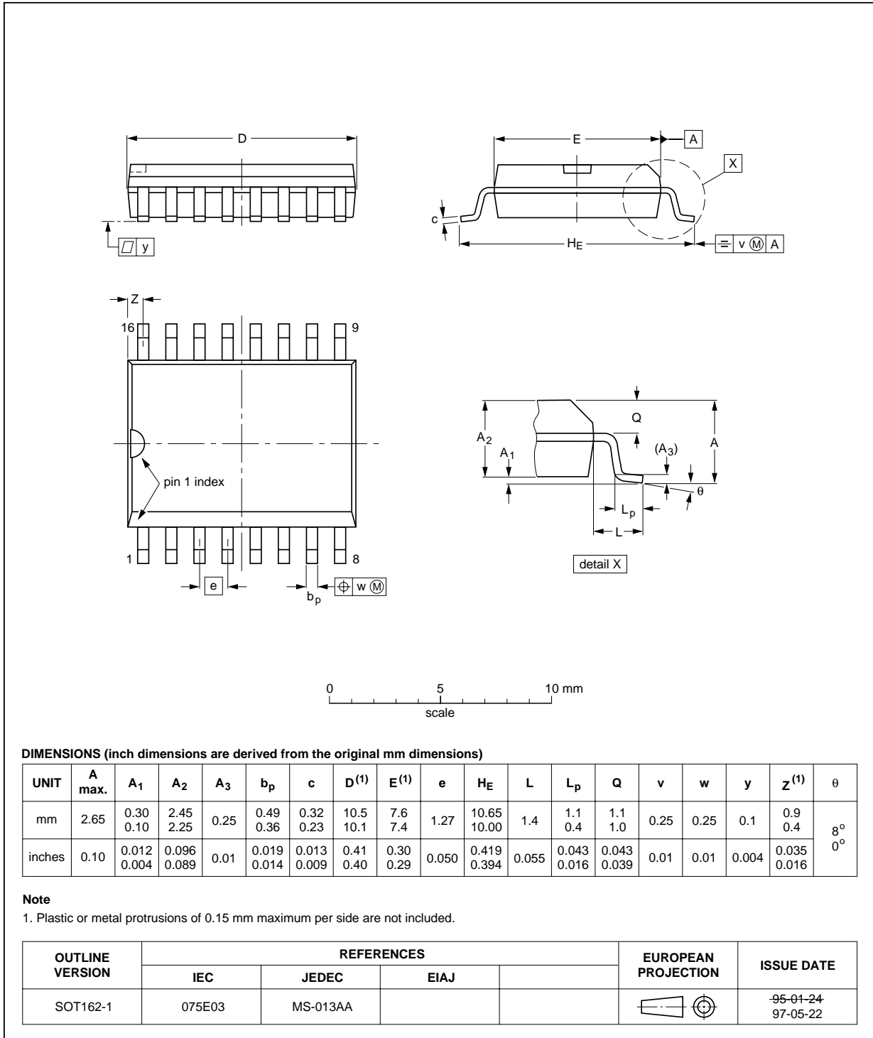
Fig 17. SOT162-1.
