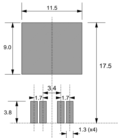
Fig.39. SOT426
