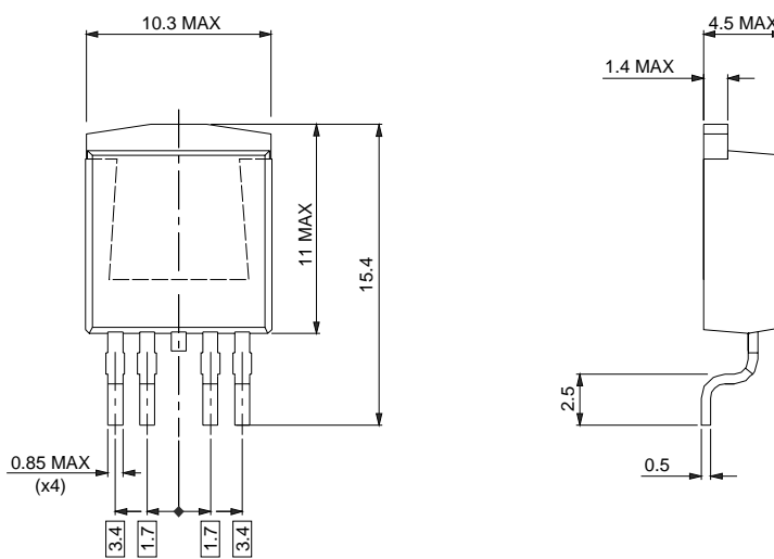
Fig.38. SOT426
