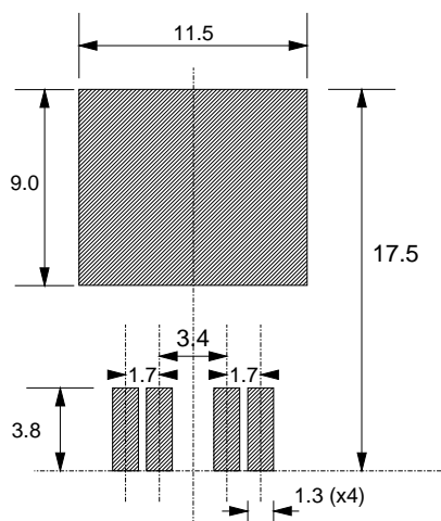
Fig.39. SOT426
